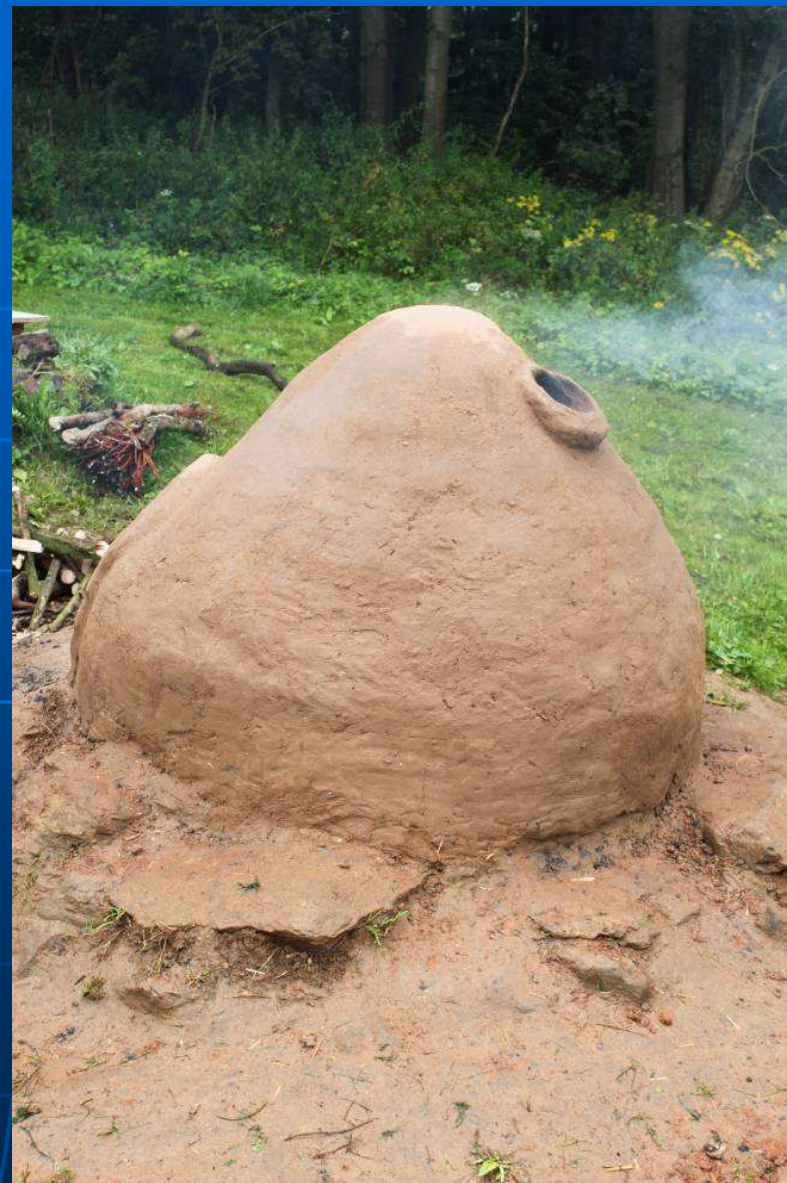
Rekostrukce chlebové pece Villa Nova Uhřínov pod Deštnou
